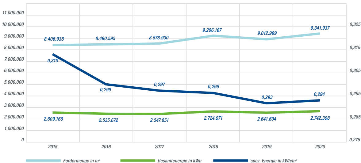
Entwicklung der spezifischen Energie der Druckerhöhungsanlagen
